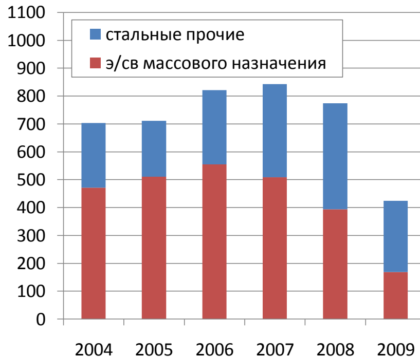
Украина: объемы потребления стальных труб, тыс. тонн
