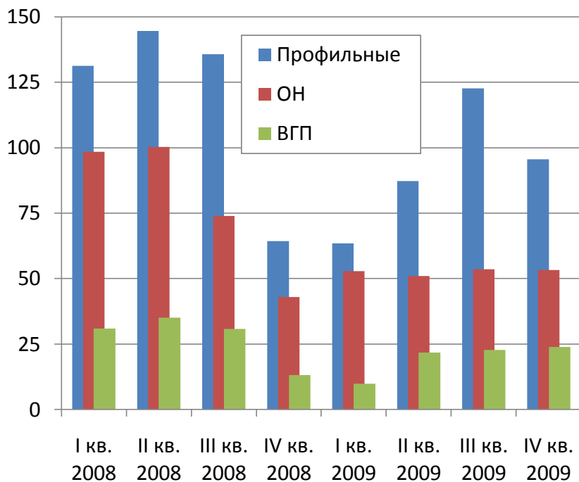
Украина: динамика производства труб МН, тыс. тонн
