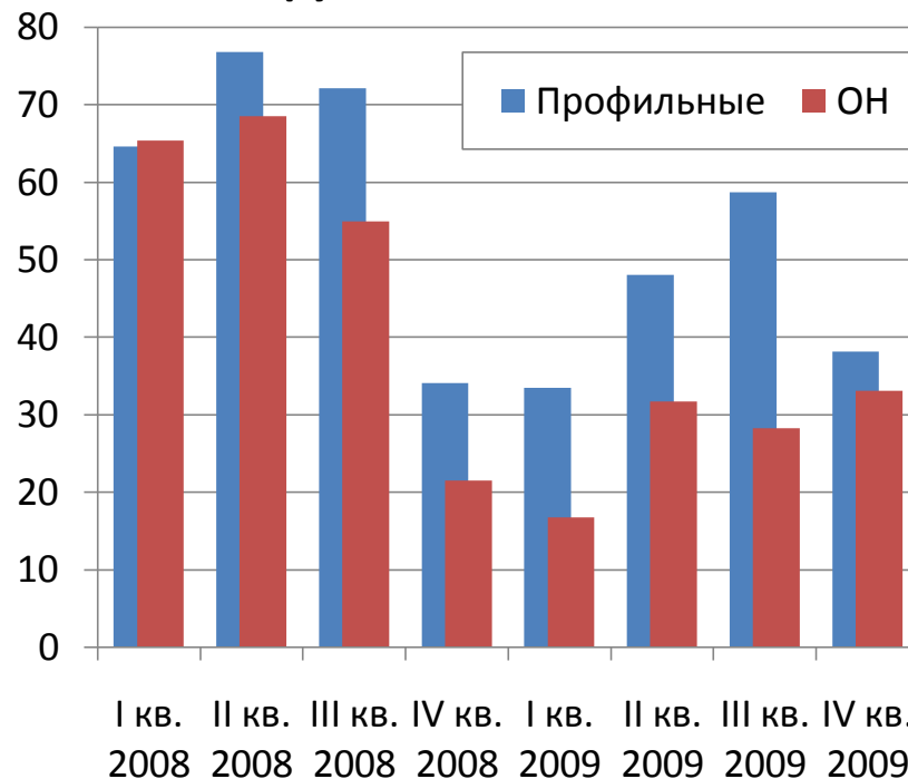
Украина: динамика потребления труб МН, тыс. тонн
