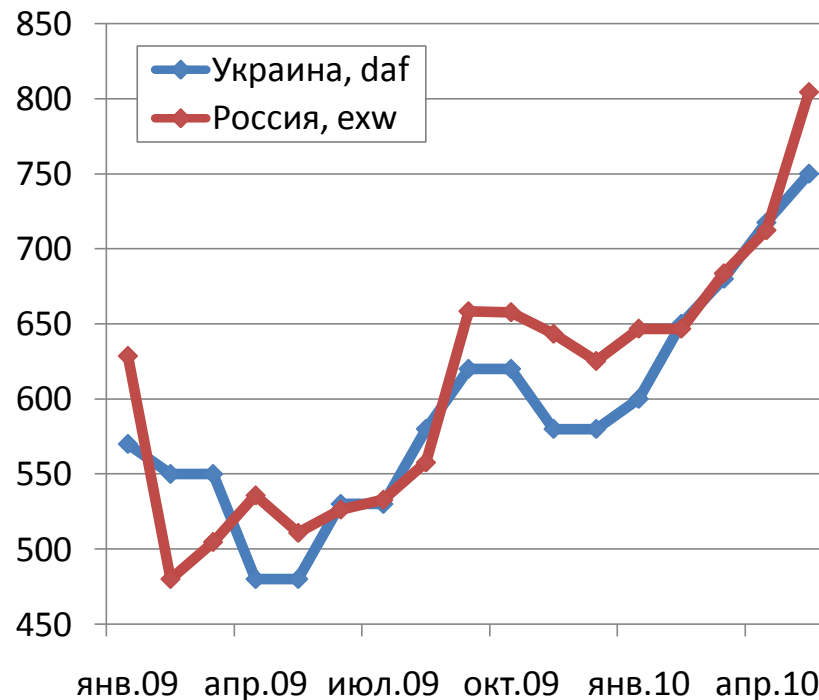
Цены производителей на э/с трубы 57-108 мм, $/т без НДС
