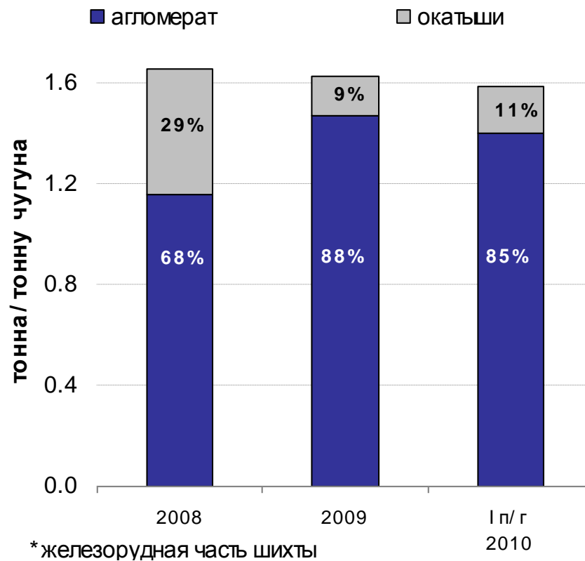
Тулачермет: структура шихты*
