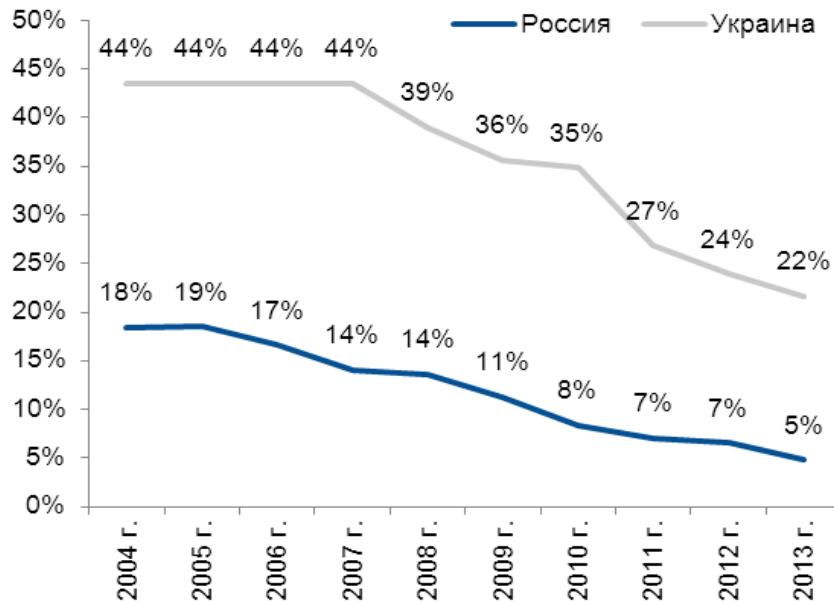
Доля мартенов в сталеплавильных мощностях
