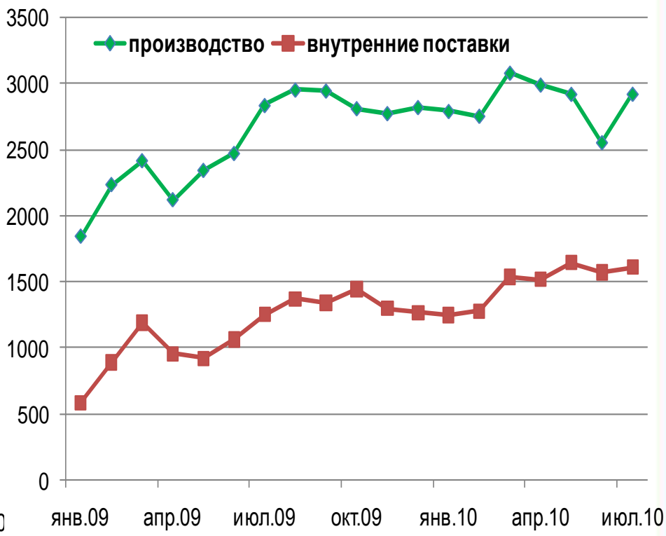
плоский прокат
